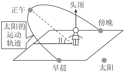
乙 正午太阳高度示意图
