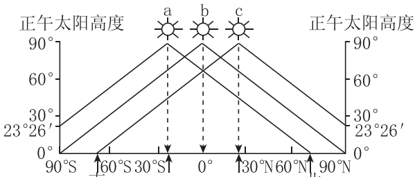
二分二至日正午太阳高度分布示意图
